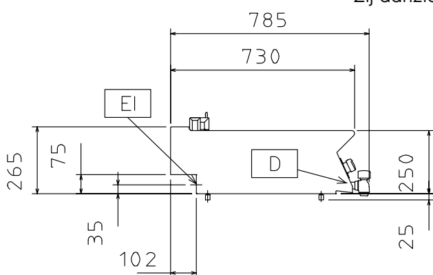
Zij aanzicht
